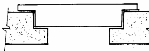
Figura 4 - Porta com sobreposição externa
